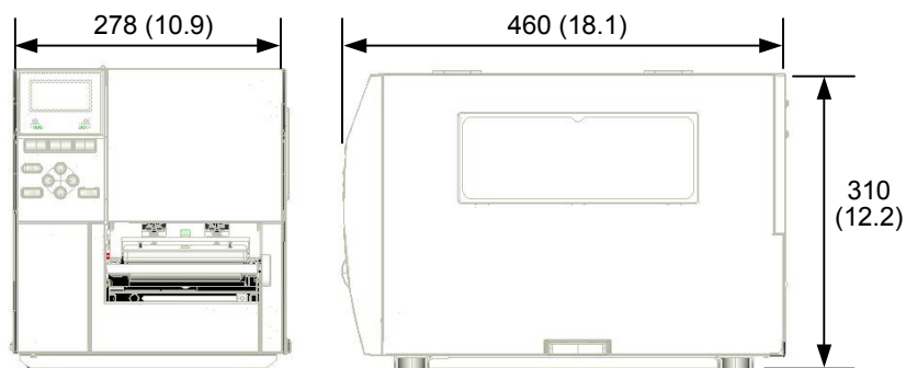
Dimensions en mm (pouces)
